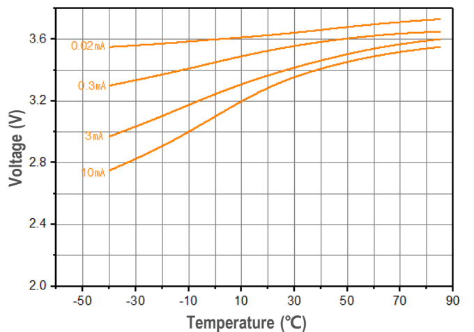
온도별 전압특성
