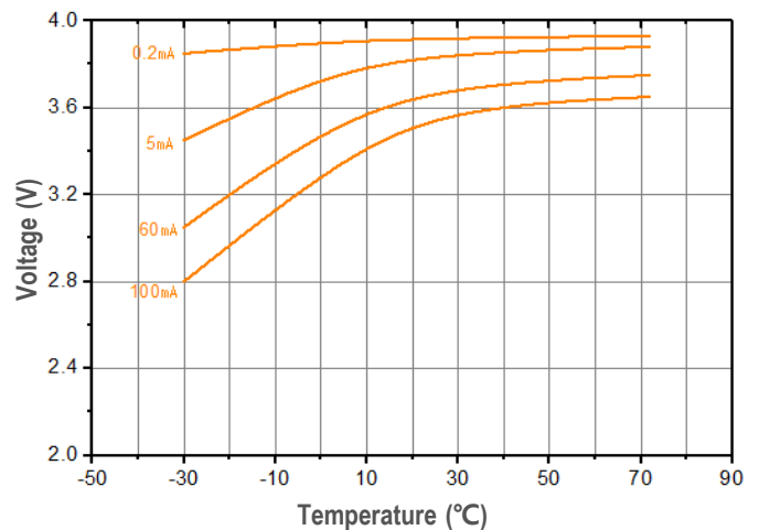
온도별 전압특성
