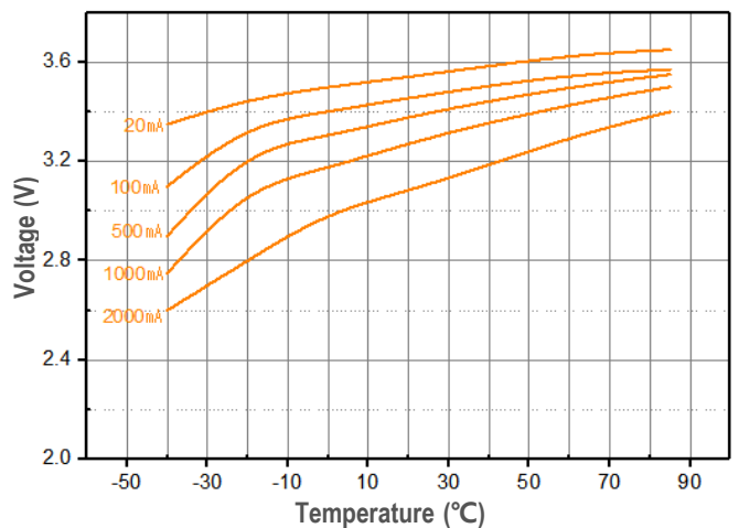
온도별 전압특성
