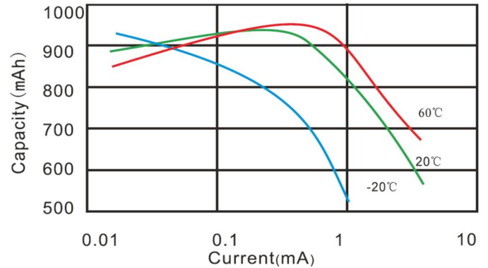
온도별 전압특성
