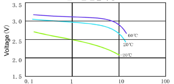
저장 및 방전특성
