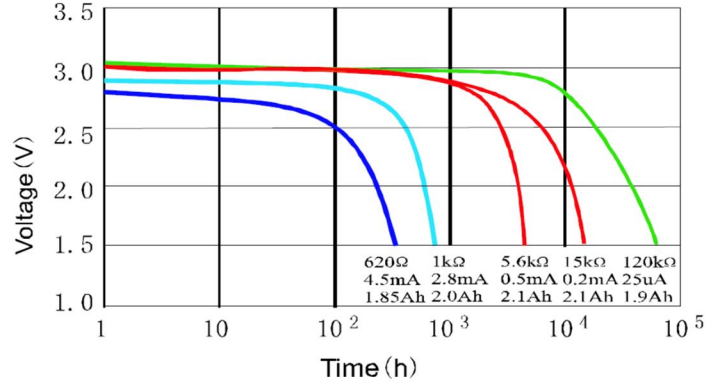
전류별 용량특성
