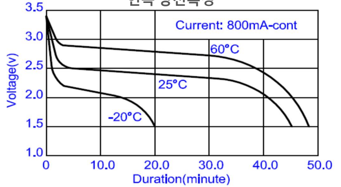
연속 방전특성
