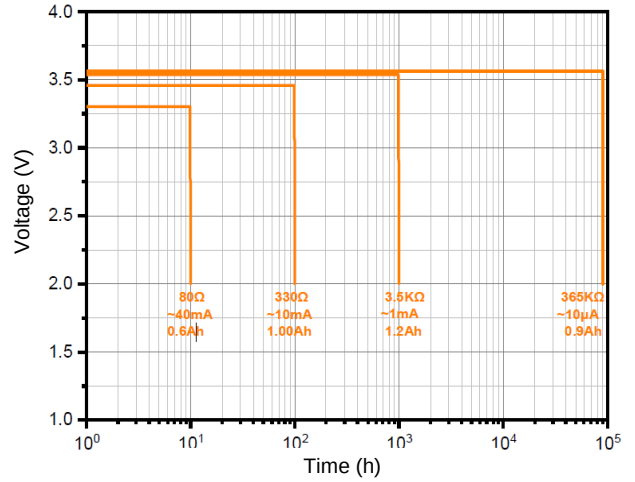
전류별 용량특성
