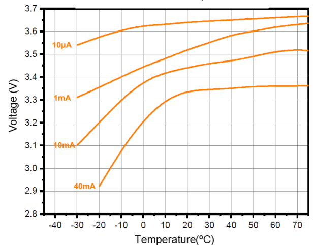
온도별 전압특성
