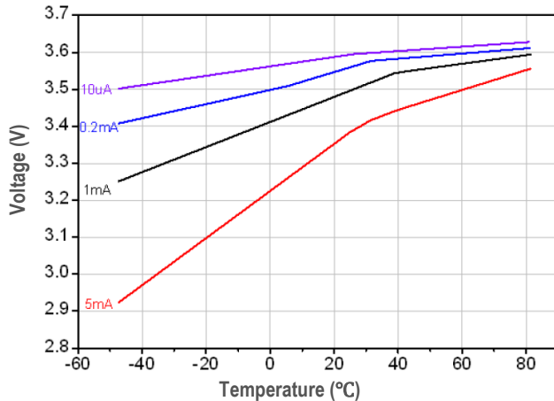
온도별 전압특성
