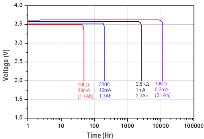
전류별 용량특성
