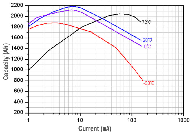
전류별 용량특성
