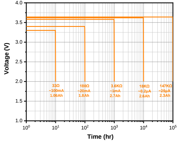
전류별 용량특성
