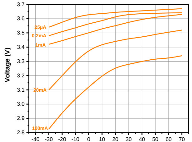
온도별 전압특성
