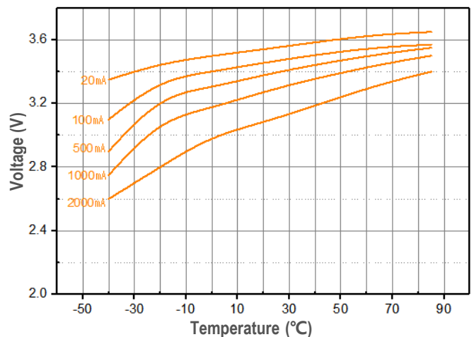
온도별 전압특성
